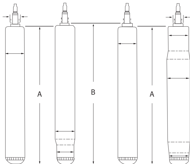
Fig. 2 Anillo-buje
