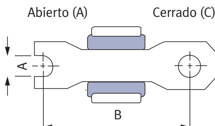
Fig. 4 Moño
