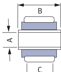
Fig. 3 Anillo-buje-camisa
